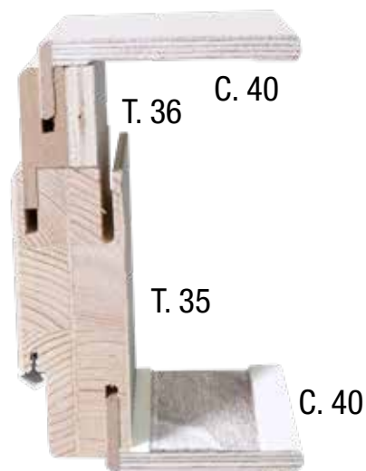
Telaio con allargamento + cornice PLUS
