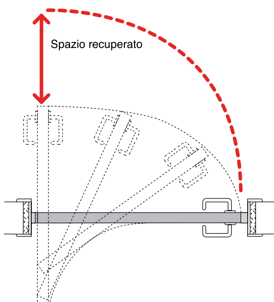
Aumenta lo spazio "Di qua - Di là - Roto"
