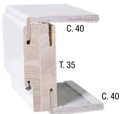
Telaio standard + cornice PLUS
